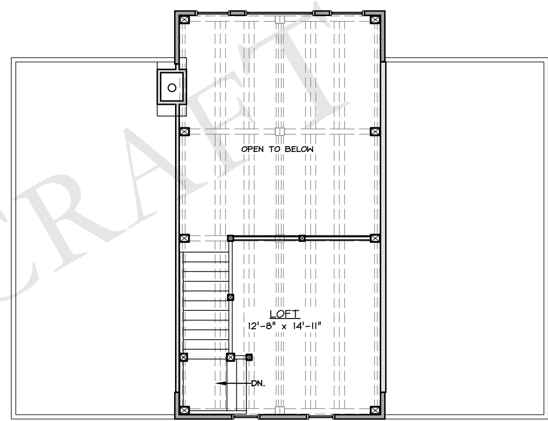
LOFT FLOOR PLAN SCALE: N.T.S.
